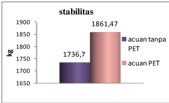
Gambar 3.7. Stabilitas campuran beton aspal tanpa dan dengan limbah botol air mineral (PET)
