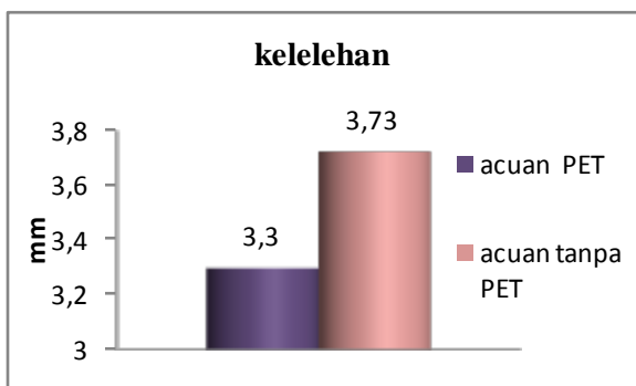
Gambar 3.9. Kelelahan campuran beton aspal tanpa dan dengan limbah botol air mineral (PET)
