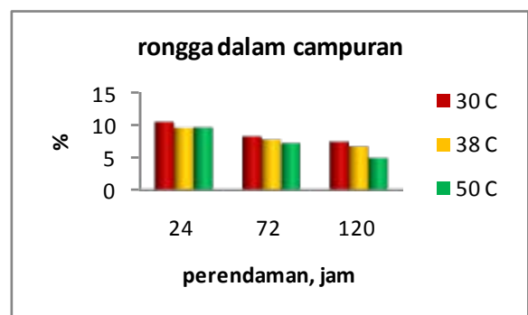
Gambar 3.6. Rongga dalam campuran beton aspal dengan limbah botol air mineral
