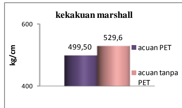
Gambar 3.11. Kekakuan campuran beton aspal tanpa dan dengan limbah botol air mineral (PET)
