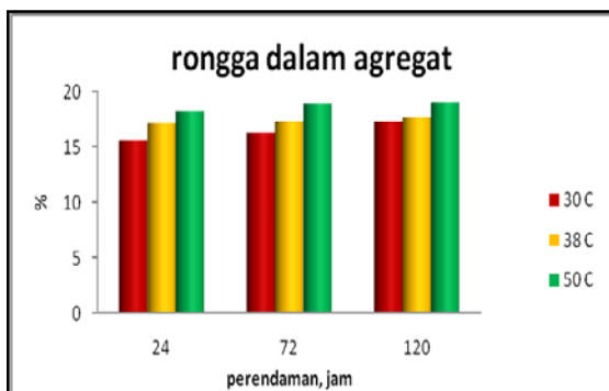
Gambar 3.4. Rongga dalam agregat campuran beton aspal dengan limbah botol air mineral
