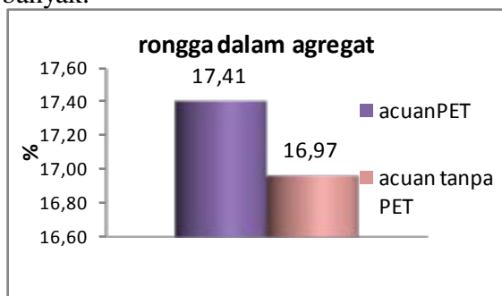
Gambar 3.3. Rongga dalam agregat beton aspal tanpa dan dengan limbah botol air mineral (PET)
