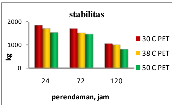
Gambar 3.8. Stabilitas campuran beton aspal dengan limbah botol air mineral
