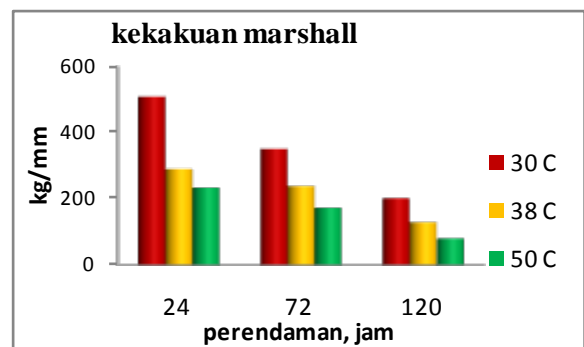
Gambar 3.12. Kekakuan campuran beton aspal dengan limbah botol air mineral
