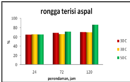
Gambar 3.2 Rongga terisi aspal campuran beton aspal dengan limbah botol air mineral
