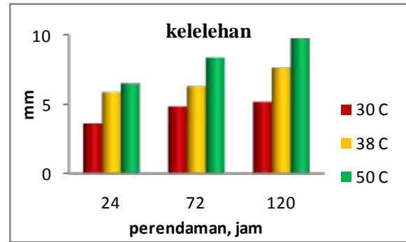
Gambar 3.10. Kelelahan campuran beton aspal dengan limbah botol air mineral
