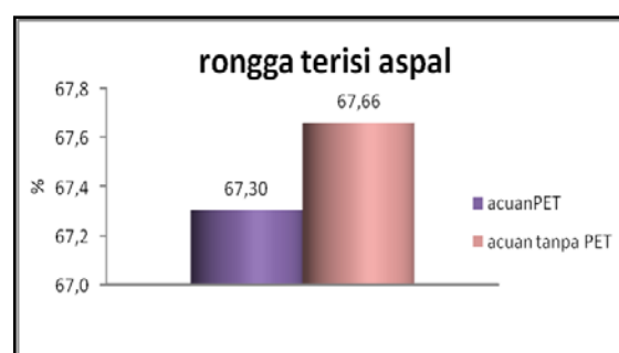
Gambar 3.1. Rongga terisi aspal beton aspal tanpa dan dengan limbah botol air mineral (PET)
