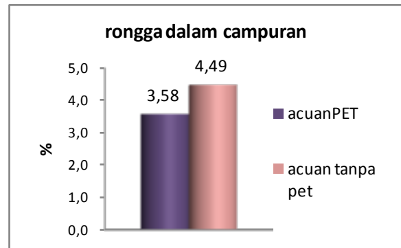
Gambar 3.5. Rongga dalam campuran beton aspal tanpa dan dengan limbah botol air mineral (PET)
