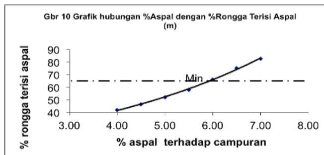
Gambar 10: Grafik hubungan % aspal dengan % rongga terisi aspal
