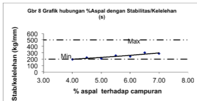
Gambar 8: Grafik hubungan % aspal dengan stabilitas/kelelehan
