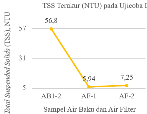
Gambar 8. Perbandingan Kualitas Air Baku dan Output Filter (TSS) pada Ujicoba I
