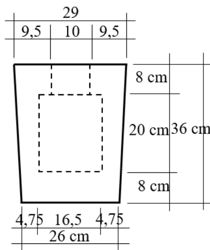
Gambar 4. Sketsa Dimensi Filter Air Cetak
