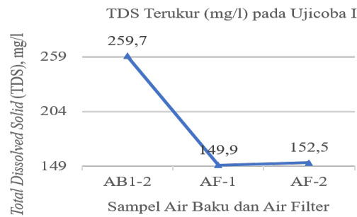
Gambar 7. Perbandingan Kualitas Air Baku dan Output Filter (TDS) pada Ujicoba I
