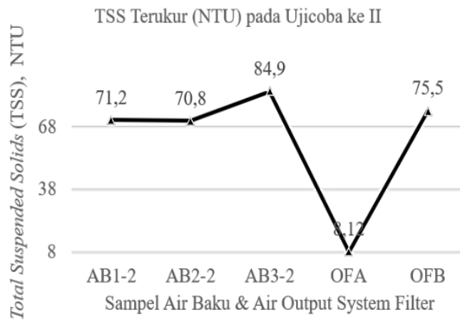
Gambar 10. Perbandingan Kualitas Air Baku dan Output System Filter (TDS) pada Ujicoba II
