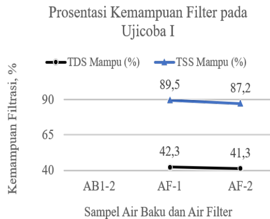
Gambar 8. Perbandingan Kualitas Air Baku dan Output Filter (TSS) pada Ujicoba I
