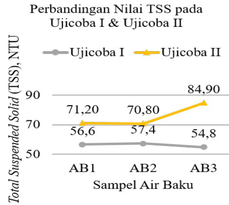
Gambar 6. Kualitas Air Baku Berdasarkan Elevasi Muka Air (TSS)
