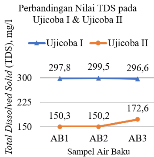
Gambar 5. Kualitas Air Baku Berdasarkan Elevasi Muka Air (TDS)
