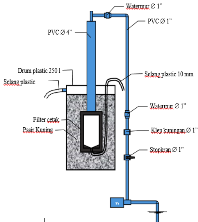
Gambar 2. Rancangan System Filter Air Cetak
