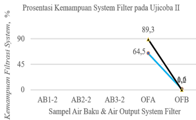
Gambar 12. Kemampuan Filter Air Cetak (System) Menurunkan Nilai TDS & TSS pada Ujicoba I
