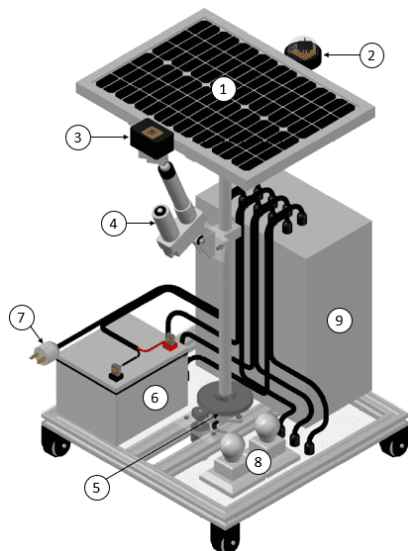
Gambar 3. Detail Komponen Pada Sistem Solar Tracker
