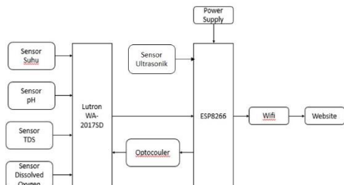
Gambar 1. Blok Diagram Sistem Monitoring Parameter Air Akuaponik
