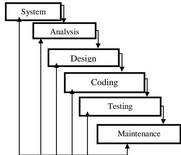
Gambar 3.2 Pengembangan Sistem
